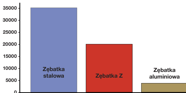
TRWAŁOŚĆ (km) ZĘBATEK SUNSTAR PRZY NORMALNEJ EKSPLOATACJI TURYSTYCZNEJ
