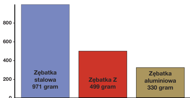
WAGA ZĘBATKI DO MOTOCYKLA BMW F650
