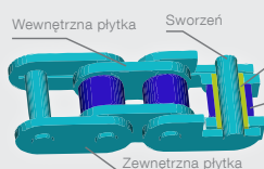
Łańcuch rolkowy
