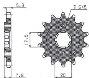
nr katalogowy 392 ilość zębów 14-15-16-17
