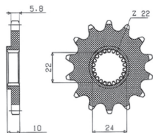
nr katalogowy 387 ilość zębów 14-15
