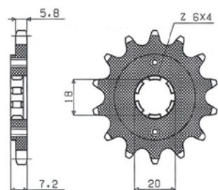
nr katalogowy 391 ilość zębów 12-13-14-15
