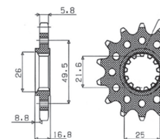
nr katalogowy 403 ilość zębów 13-14-15
