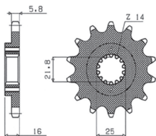
nr katalogowy 389 ilość zębów 14-15
