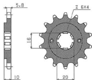
nr katalogowy 386 ilość zębów 15-16
