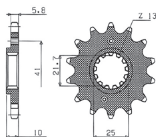
nr katalogowy 388 ilość zębów 12-13-14-16
