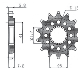
nr katalogowy 397 ilość zębów 13-14-15-16-17
