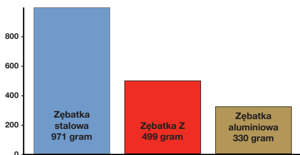
WAGA ZĘBATKI DO MOTOCYKLA BMW F650
