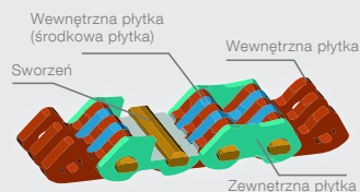
Łańcuch płytkowy (cichy)
